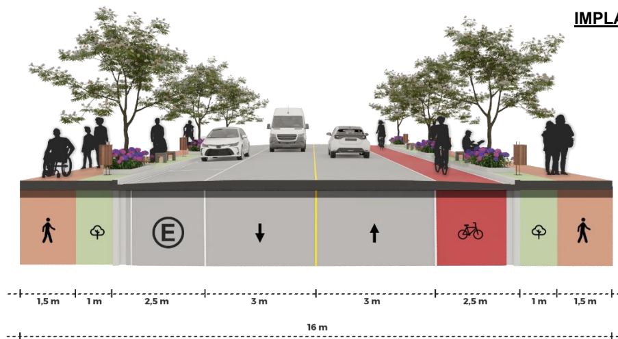
SECÇÃO TRANSVERSAL
