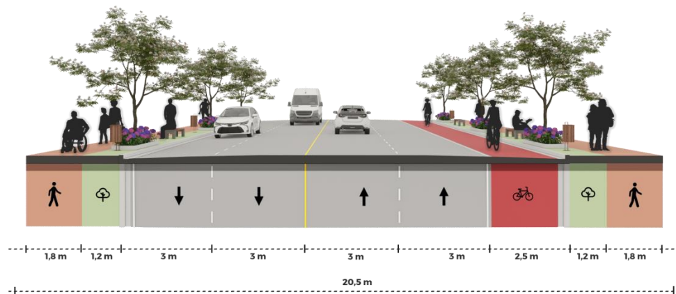
SECÇÃO TRANSVERSAL
